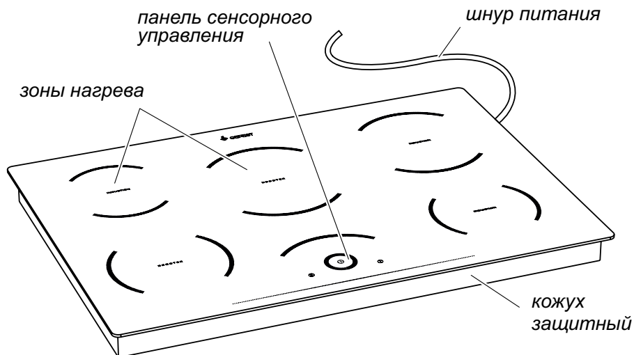
Рис. 1 Панель варочная
